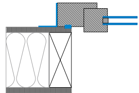
> Alternative mit Fugendichtband oder Rundschnur
