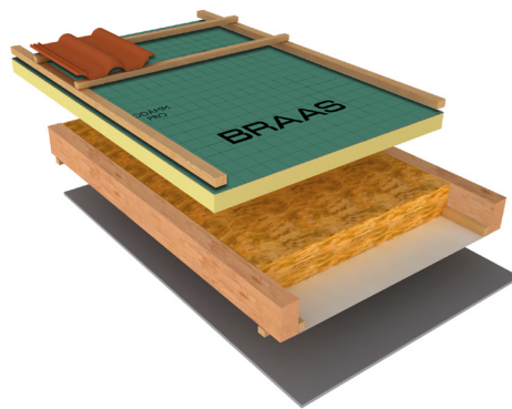
Kombination von Mineralwolle mit DivoDämm und DivoDämm Membran 2 2S.
