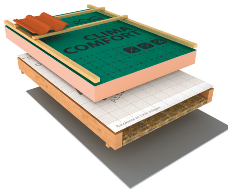
Kombination von Mineralwolle mit Clima Comfort und DivoDämm Membran 2 2S.
