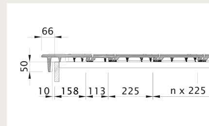
Ortgangausbildung mit Ortgangziegel links mit Ortgangbrett
