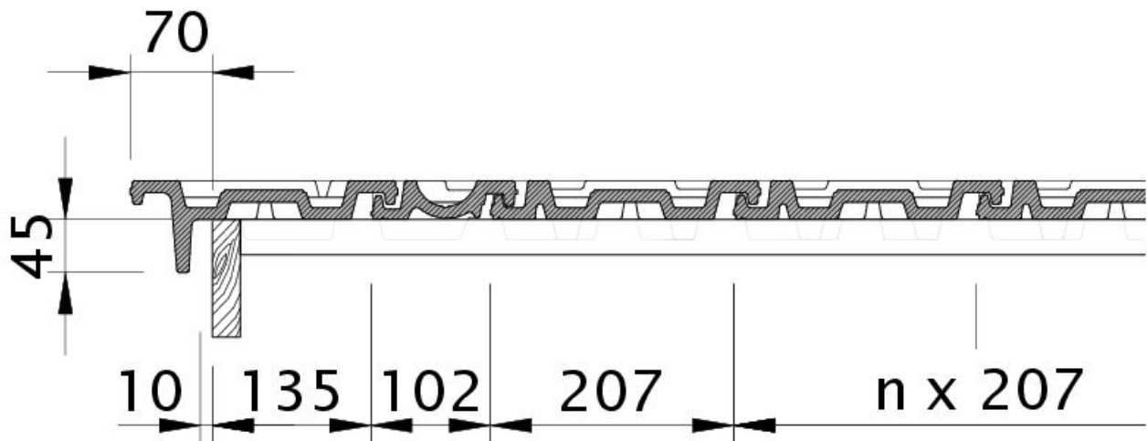
Zeichnung HERZZIEGEL Gesamtansicht GES
