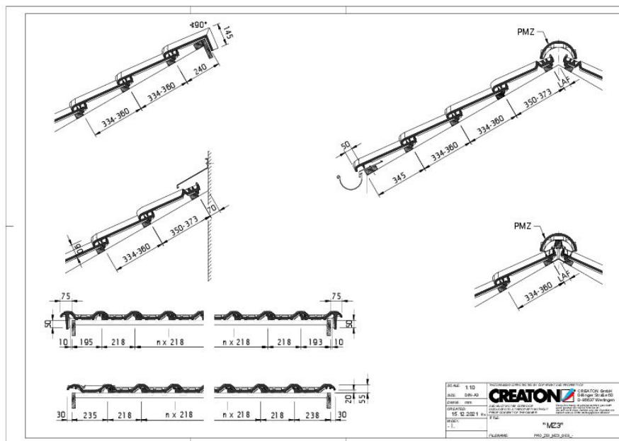
Zeichnung MZ3 NEU Gesamtansicht GES
