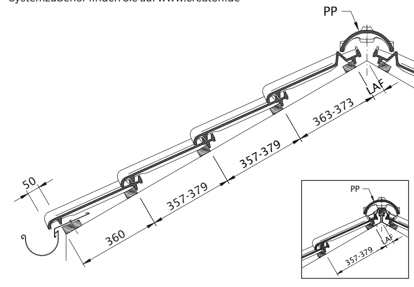
Pulldach-Ausführung
