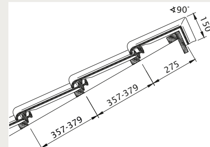
Pulldach-Ausführung
