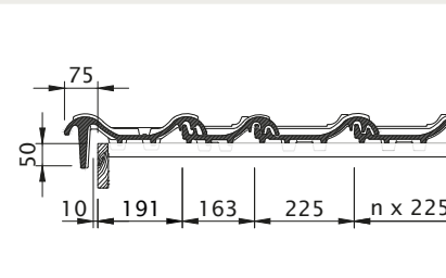
Ortgangausbildung mit Ortgangziegel links mit Ortgangbrett
