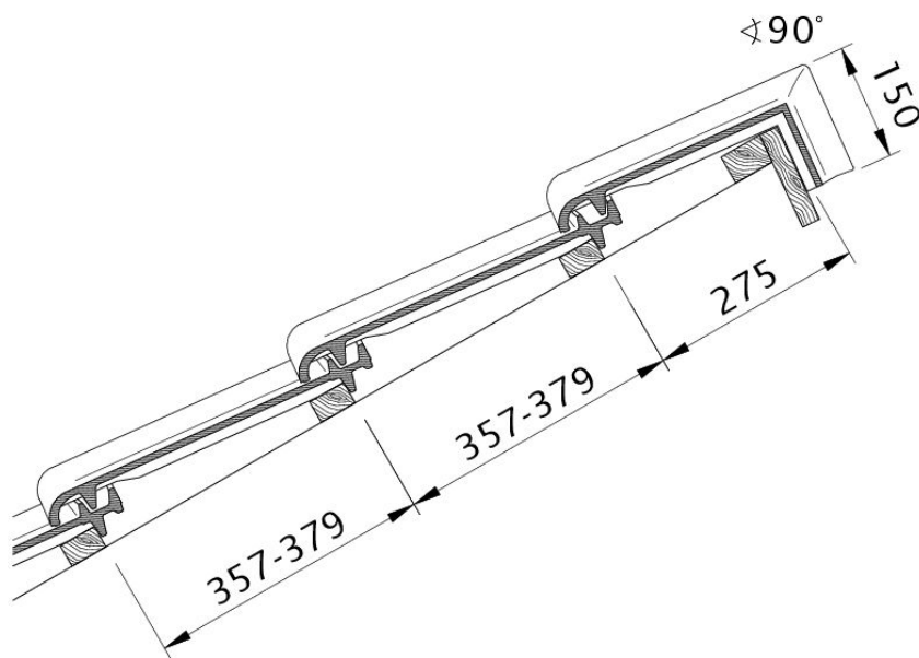
Zeichnung PREMION Pulldach-Ausführung PDA
