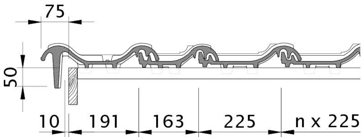
Zeichnung PREMION Dachquerschnitt DQF
