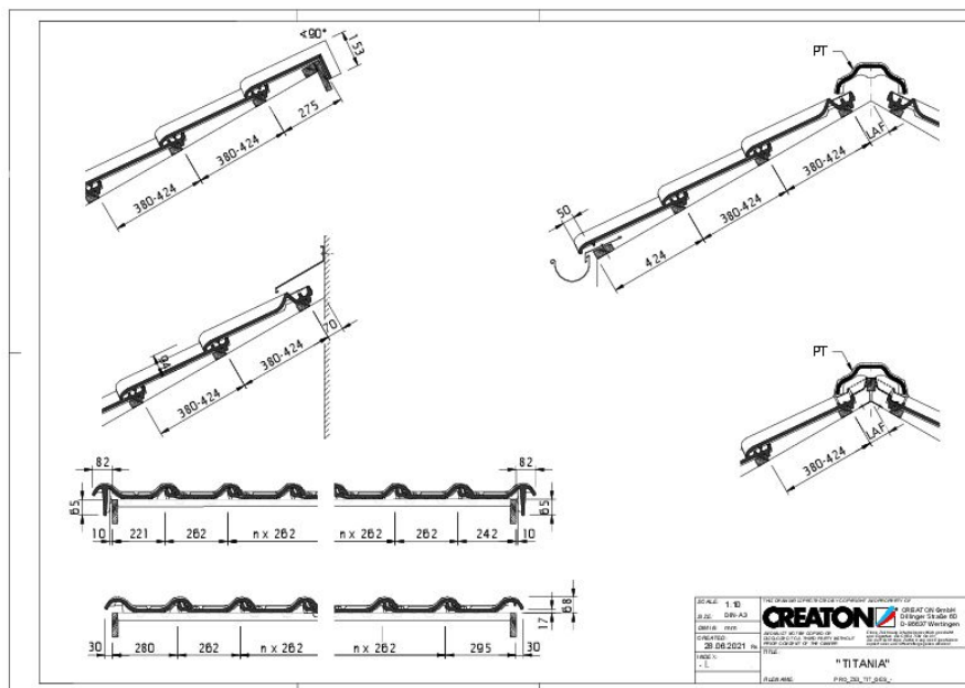
Zeichnung TITANIA Gesamtansicht GES
