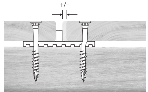
BASO reduziert die Abscherkkräfte um 50% ✓
