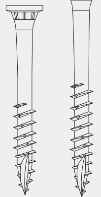
Fassadenschraube Ø 4,5 mm
