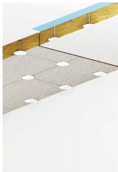
Dübelmontage / Klebe- und Dübelmontage Seite 10
