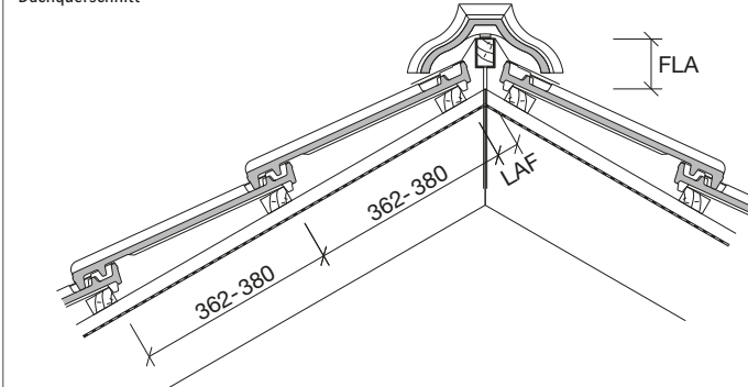
Dachquerschnitt**
