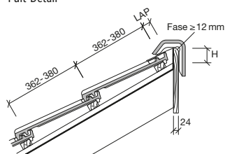
Pult-Detail**
