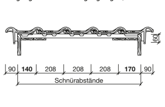
Ortgang - Detail mit Ortgangziegel*/**
