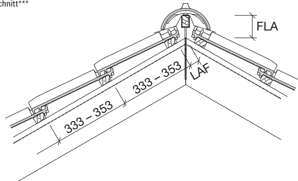
Dachquerschnitt***
