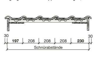
Ortgang - Detail mit Doppelwulstziegel*/**
