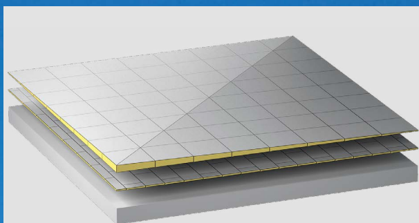
LINITHERM PAL Gefälledämmung mit Gratplatten von 230 mm bis 30 mm, für besseren U-Wert mit vollflächiger Unterlage bei Rinnenentwässerung
