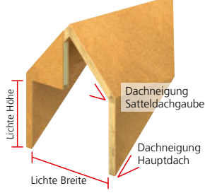
Satteldachgaube
