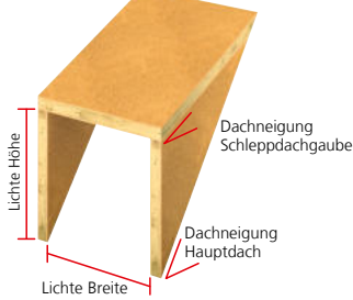
Schleppgaube
