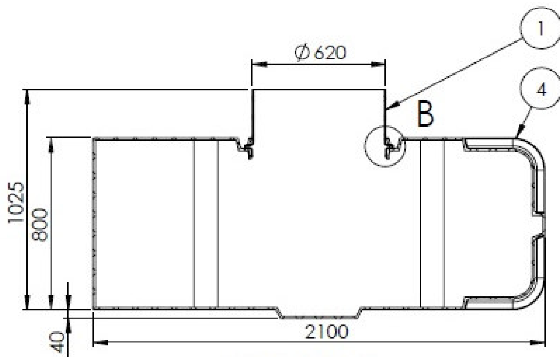
SCHNITT A-A
