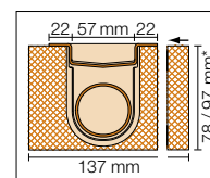
Querschnitt Mitteleinbau
