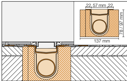
Schlüter®-KERDI-LINE-H (Miteleinbau)
