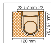
Querschnitt Wandeinbau
