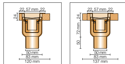
Querschnitt Wandeinbau
