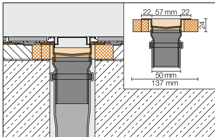
Schlüter®-KERDI-LINE-V GSE (Miteleinbau)
