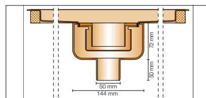
Längsschnitt Wand- / Mitteleinbau
