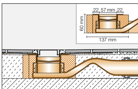
Schlüter®-KERDI-LINE-F (Miteleinbau)
