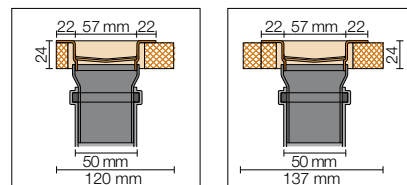
Querschnitt Wandeinbau
