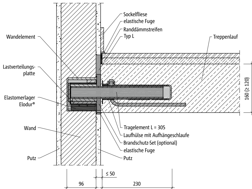
Abb. 83: Schöck Tronsole® Typ Q-FV oder Q-A2: Einbauschnitt Wanddicke 11,5 cm
