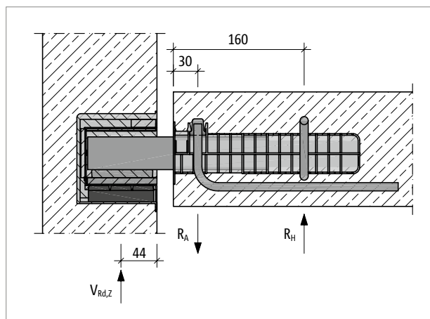
Abb. 96: Schöck Tronsole® Typ Q: statisches System
