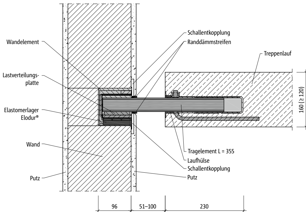
Abb. 84: Schöck Tronsole® Typ Q-FV-XL oder Q-A2-XL: Einbauschnitt
