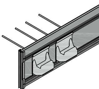
Abb. 107: Schöck Tronsole® Typ T : Detail Tragkonsole positive Fertigung
