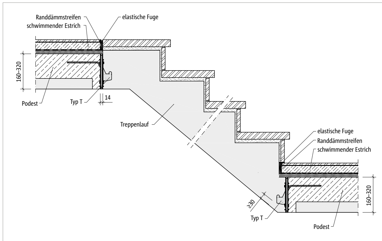
Abb. 110: Schöck Tronsole® Typ T: Einbauschnitt Fertigteiltreppe mit Halbfertigteilpodest
