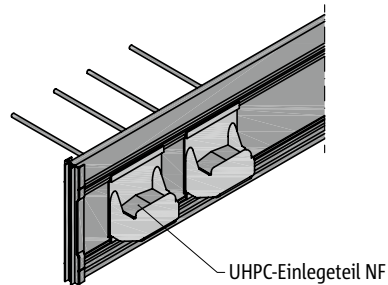
Abb. 108: Schöck Tronsole® Typ T : Detail Tragkonsole negative Fertigung
