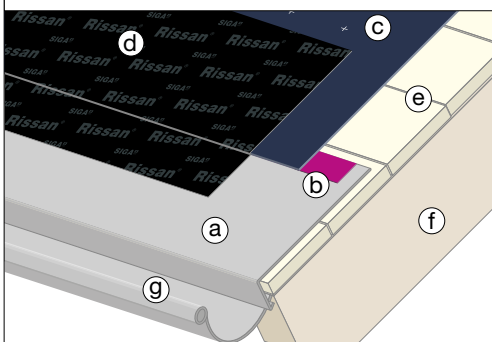
Traufanschluss für Dachneigung ab 5°
