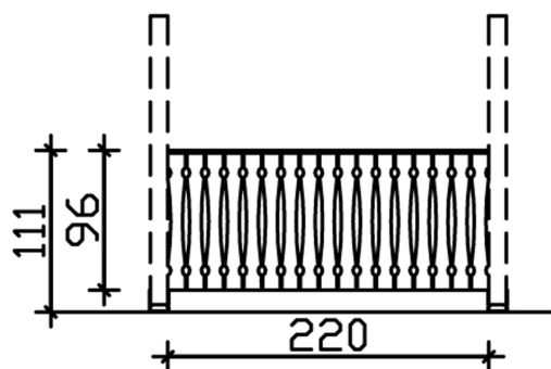
Bemassung
