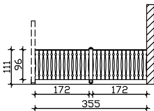
Bemassung
