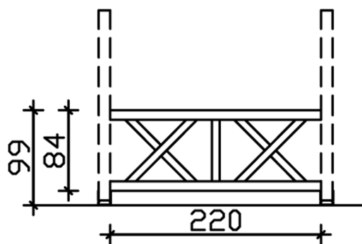
Bemassung
