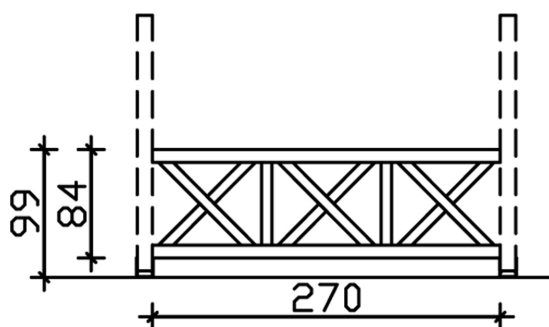
Bemassung
