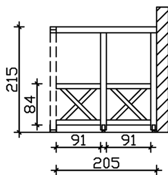
Bemassung
