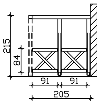
Bemassung
