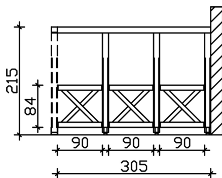
Bemassung
