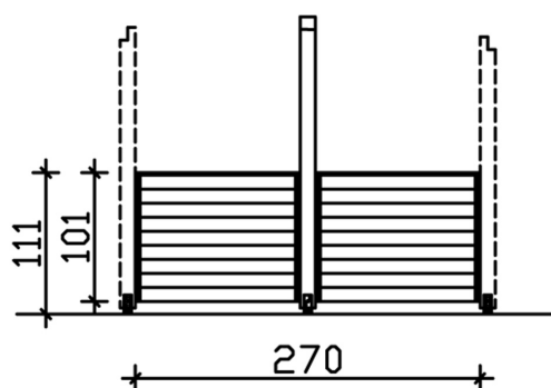
Bemassung
