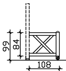
Bemassung
