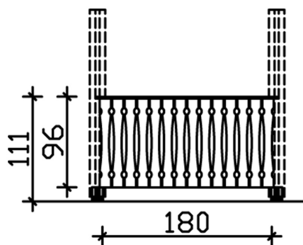
Bemassung
