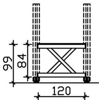
Bemassung
