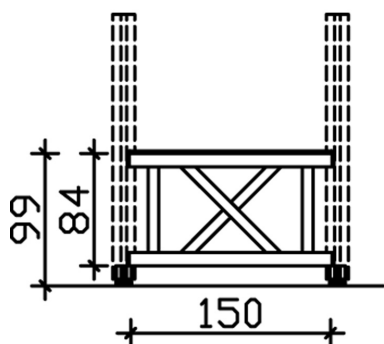
Bemassung
