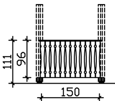
Bemassung
