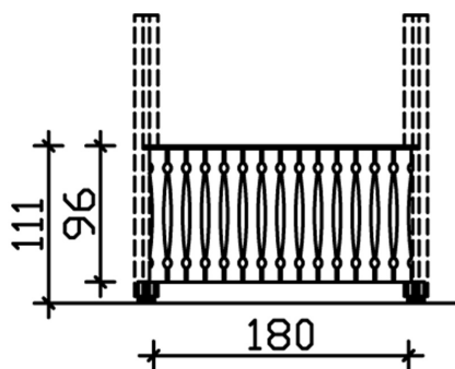
Bemassung
