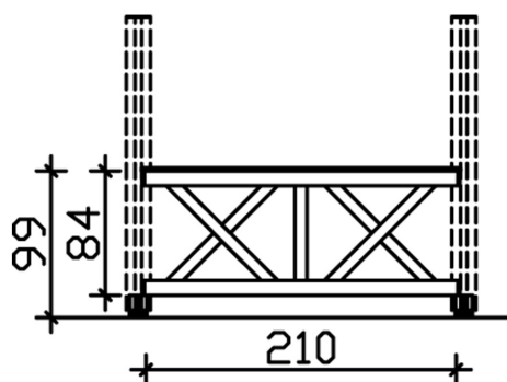
Bemassung
