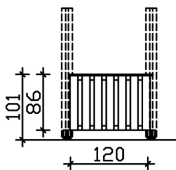
Bemassung
