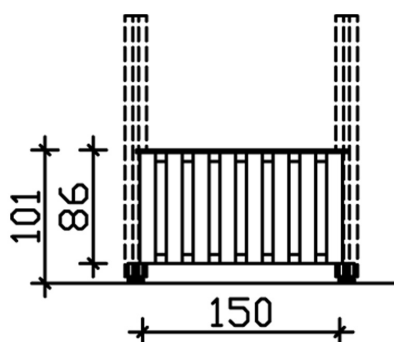
Bemassung
