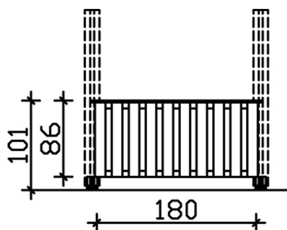
Bemassung
