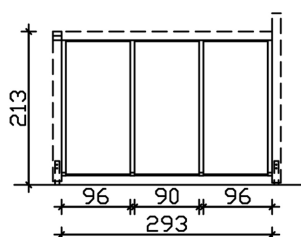
Bemassung
