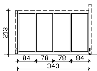
Bemassung
