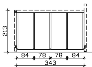
Bemassung
