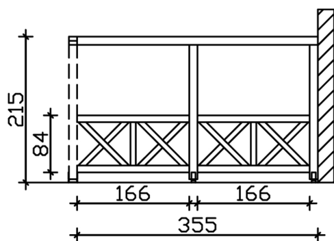
Bemassung
