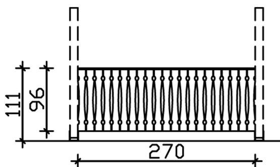
Bemassung
