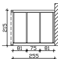
Bemassung
