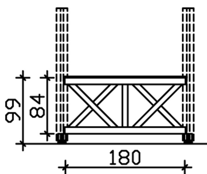
Bemassung
