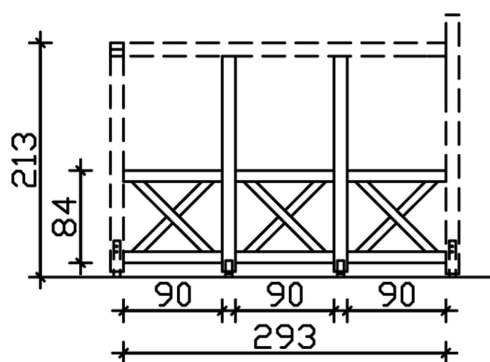
Bemassung
