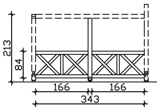
Bemassung
