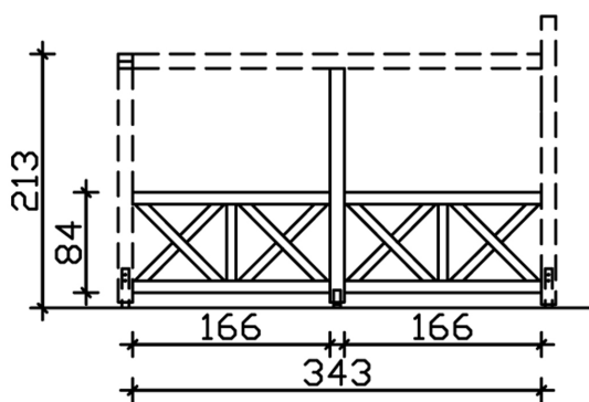
Bemassung
