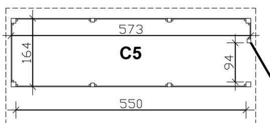
Grundriss Abstellraum C5
