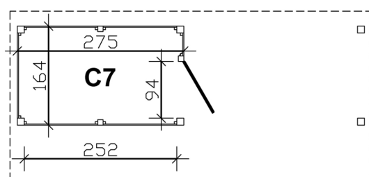
Grundriss Abstellraum C7
